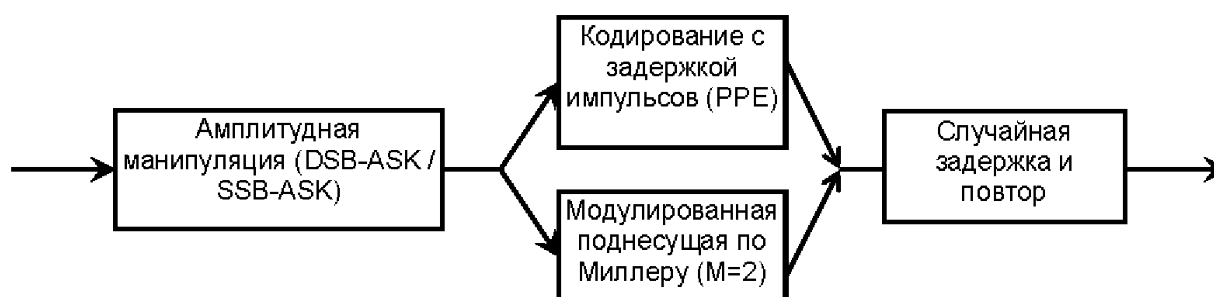
Рисунок 8 — Структура радиочастотной метки типа D
