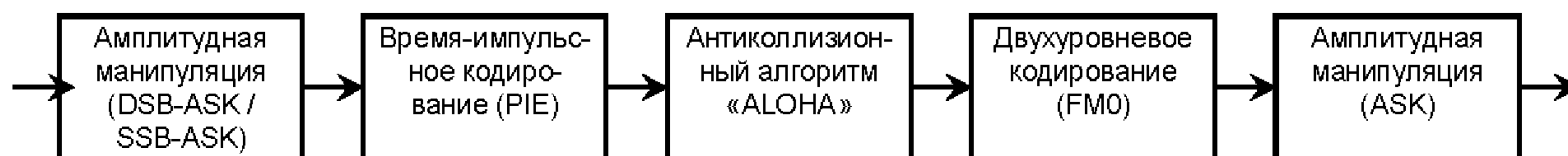
Рисунок 5 — Структура радиочастотной метки типа А
