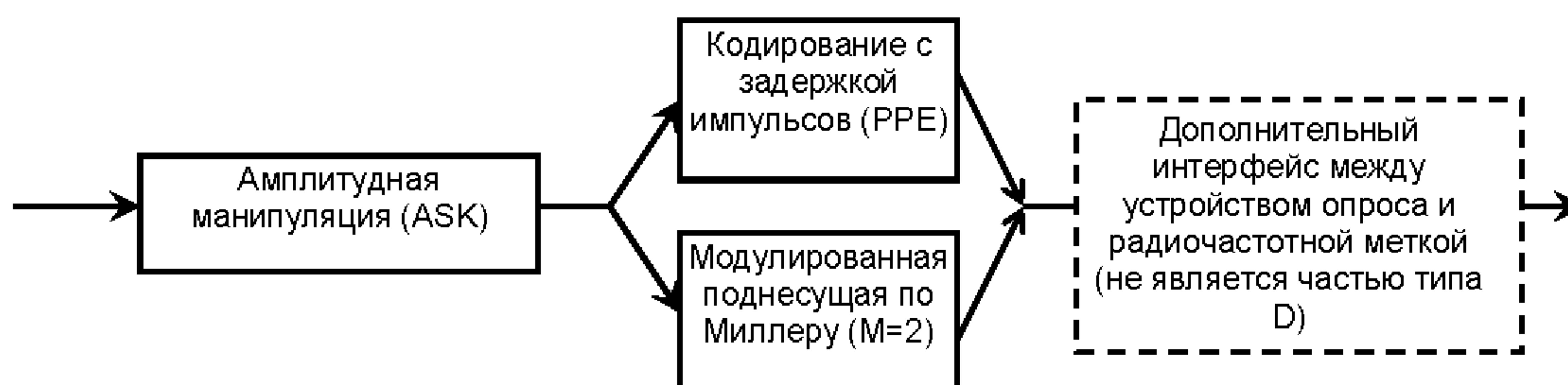
Рисунок 4 — Структура устройства опроса типа D
