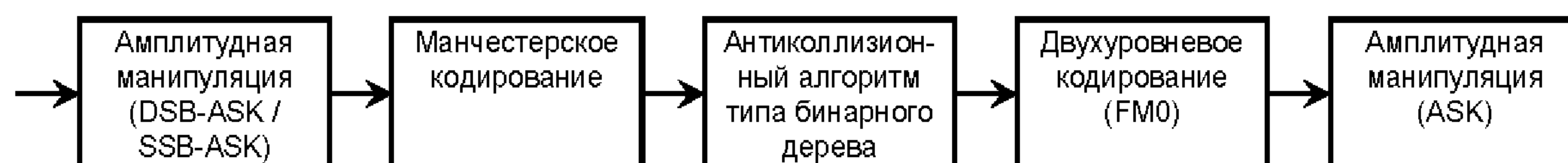
Рисунок 6 — Структура радиочастотной метки типа В
