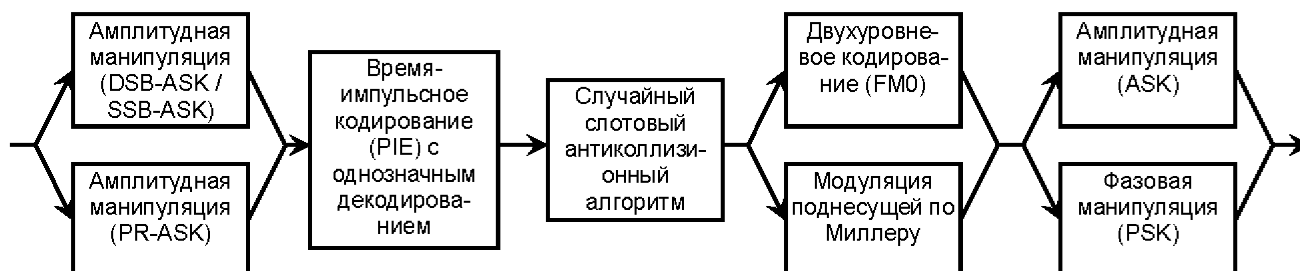
Рисунок 7 — Структура радиочастотной метки типа С
