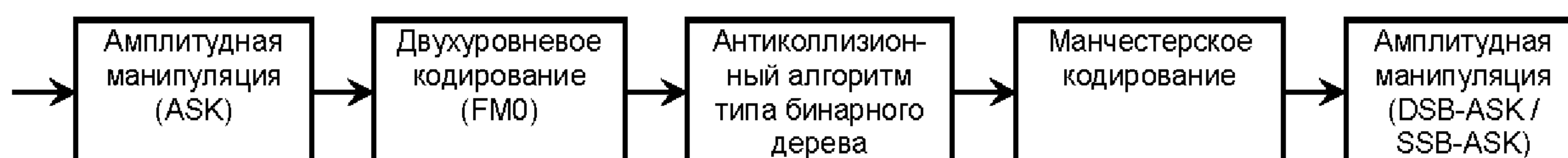
Рисунок 2 — Структура устройства опроса типа В
