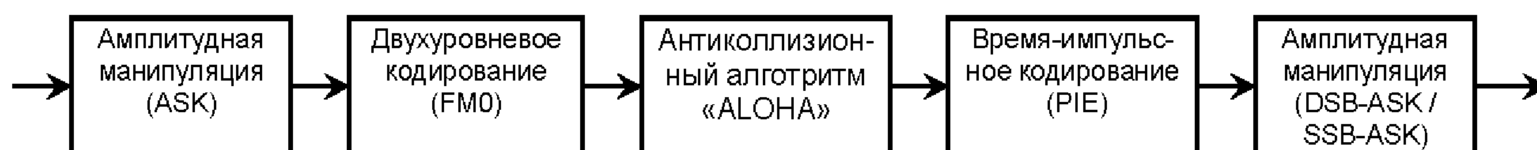
Рисунок 1 — Структура устройства опроса типа А
