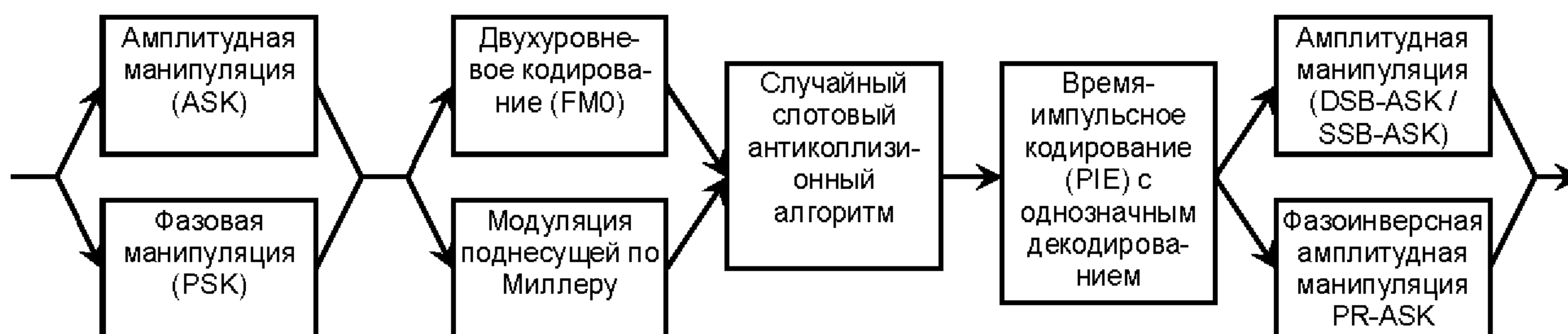
Рисунок 3 — Структура устройства опроса типа С
