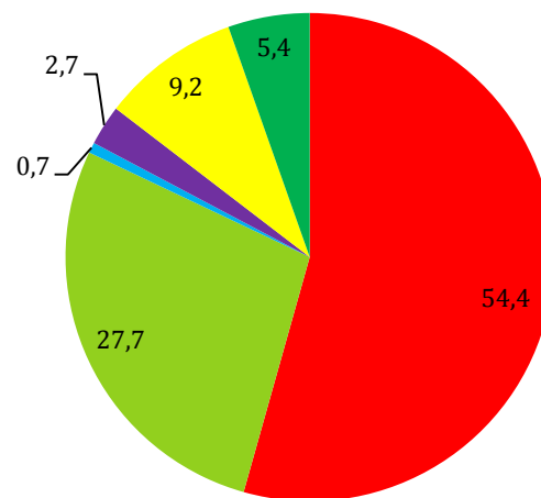
б) Казахстан
