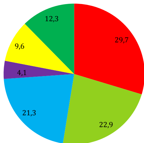
а) Беларусь
