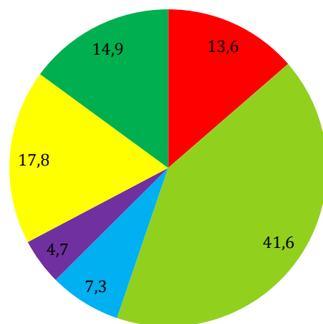
в) Россия
