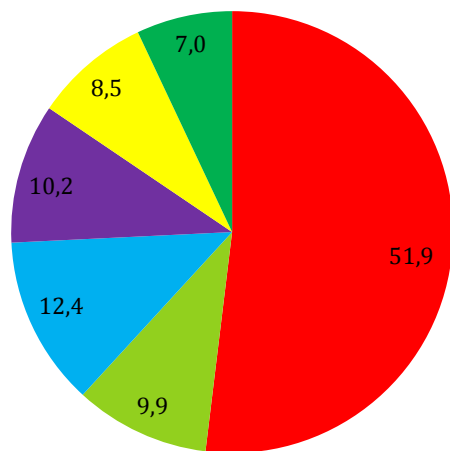
а) Беларусь
