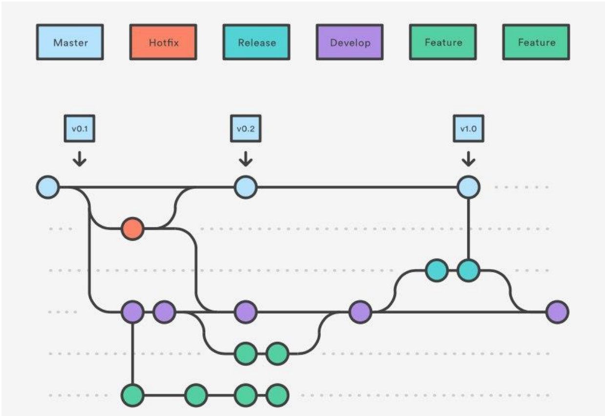
Рисунок 1 – Модель ветвления GitFlow
