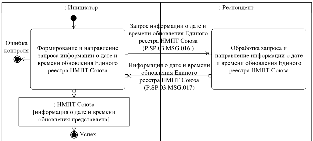
Рис. 12. Схема выполнения транзакции общего процесса «Получение информации о дате и времени последнего обновления Единого реестра НМПТ Союза» (P.SP.03.TRN.008)
