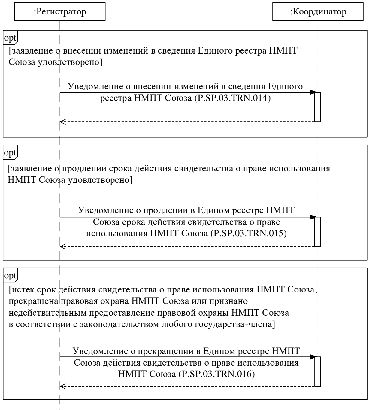
Рис. 3. Схема выполнения транзакций общего процесса при внесении изменений в сведения Единого реестра НМПТ Союза
