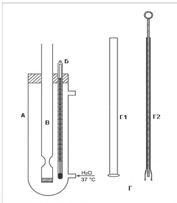
Рисунок 2.1.9.11.-2. — Прибор 2. А — водяная баня; В — термометр; В — стеклянная трубка; Г1 — стеклянный стержень; Г2 — проникающая вставка
