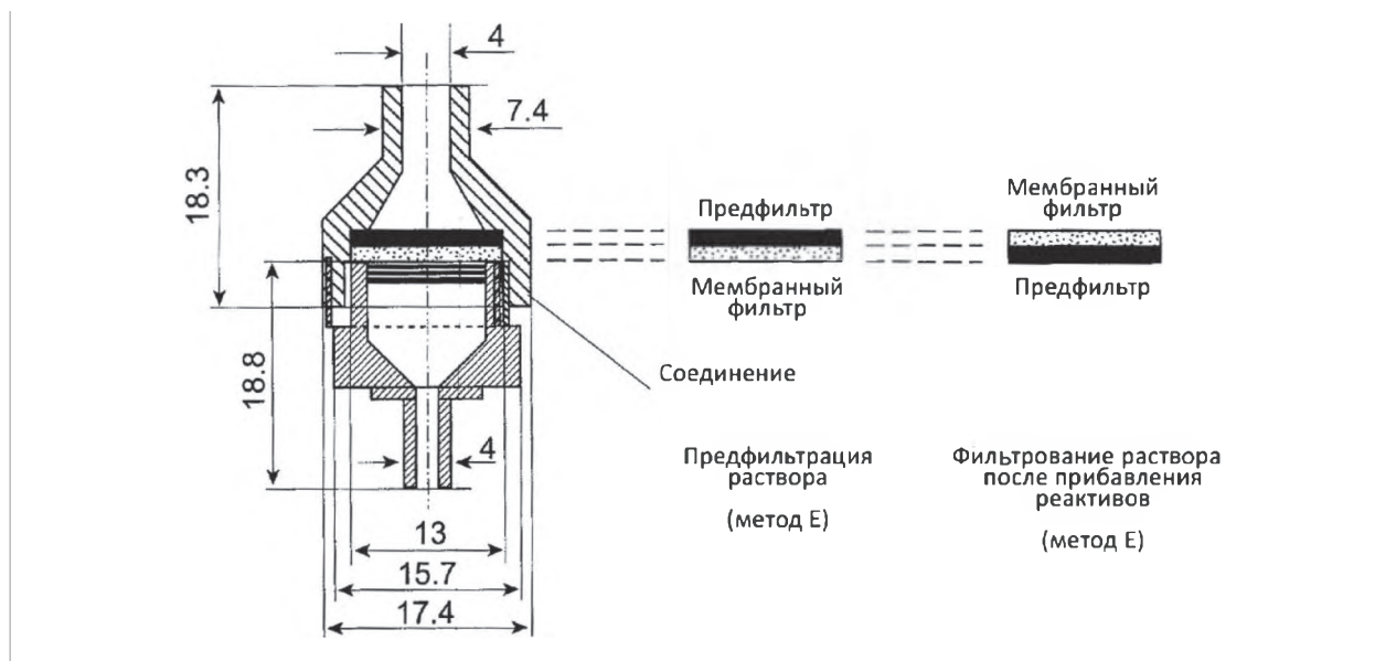
Рисунок 2.1.4.8.-1. — Прибор для испытания на соли тяжелых металлов (размеры в миллиметрах)
