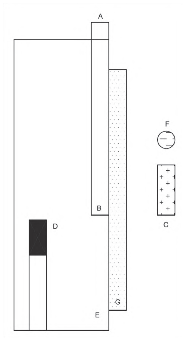
Рисунок 2.1.2.42.-2. — Способ В — отражение. А. Стекло́нная капилля́рная трубка; В. Испытуе́мый образец; С. Датчик изображе́ния; D. Температу́рный датчик; E. Нагрева́тельный блок; F. Исто́чник света; G. Прозра́чная пластинка.
