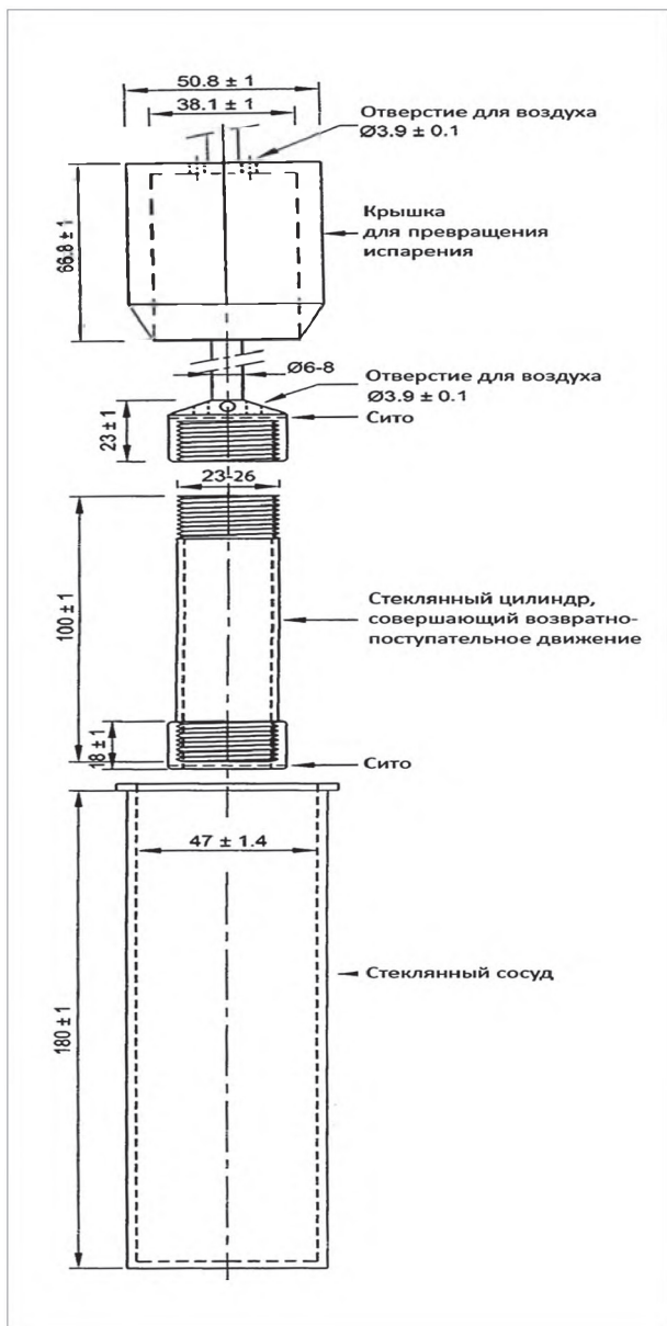
Рисунок 2.1.9.3.-4. — Прибор 3, стекло́нный сосуд и пори́невый цилиндр (размеры в миллиметрах при отсутствии других указаний)
