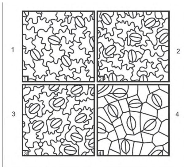
Рисунок 2.1.8.3.-1. — Типы устьиц.
