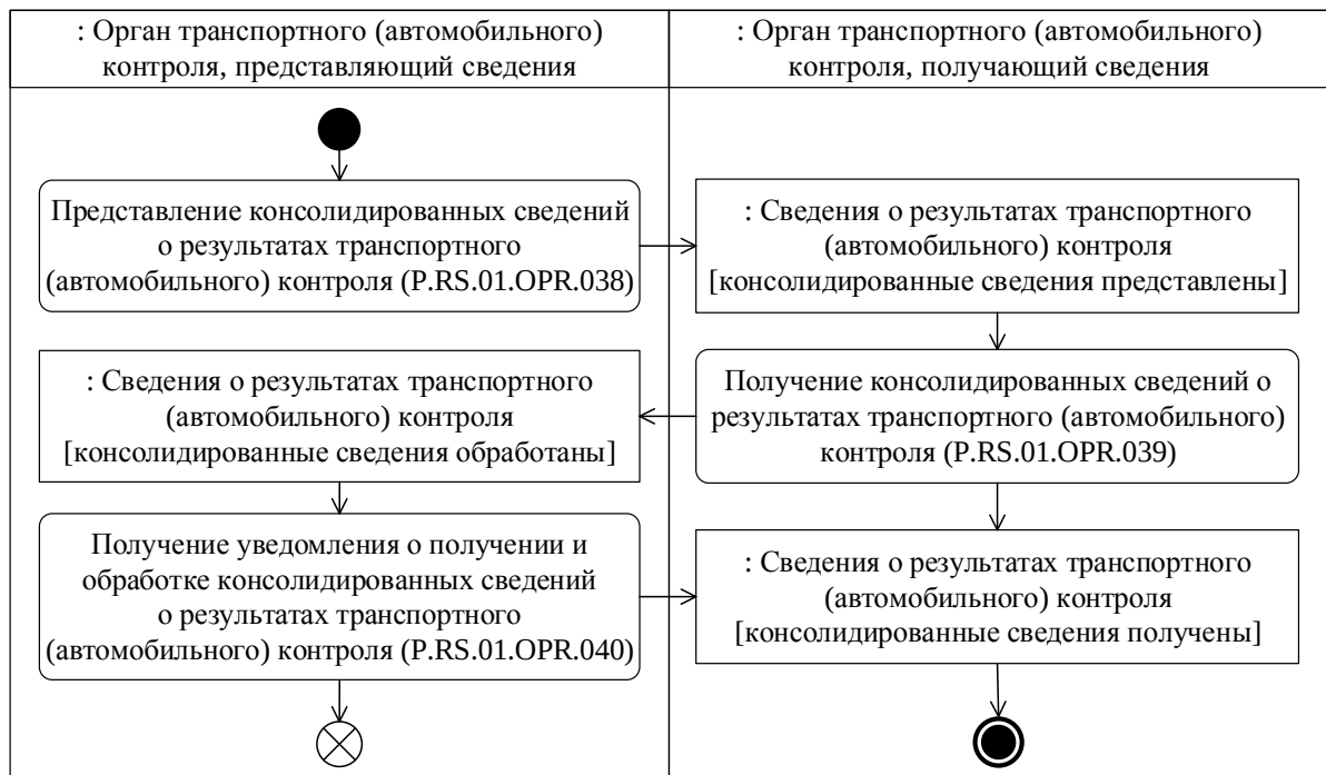
Рис. 8. Схема выполнения процедуры «Учет, хранение и передача консолидированных сведений о результатах транспортного (автомобильного) контроля» (P.RS.01.PRC.004)
