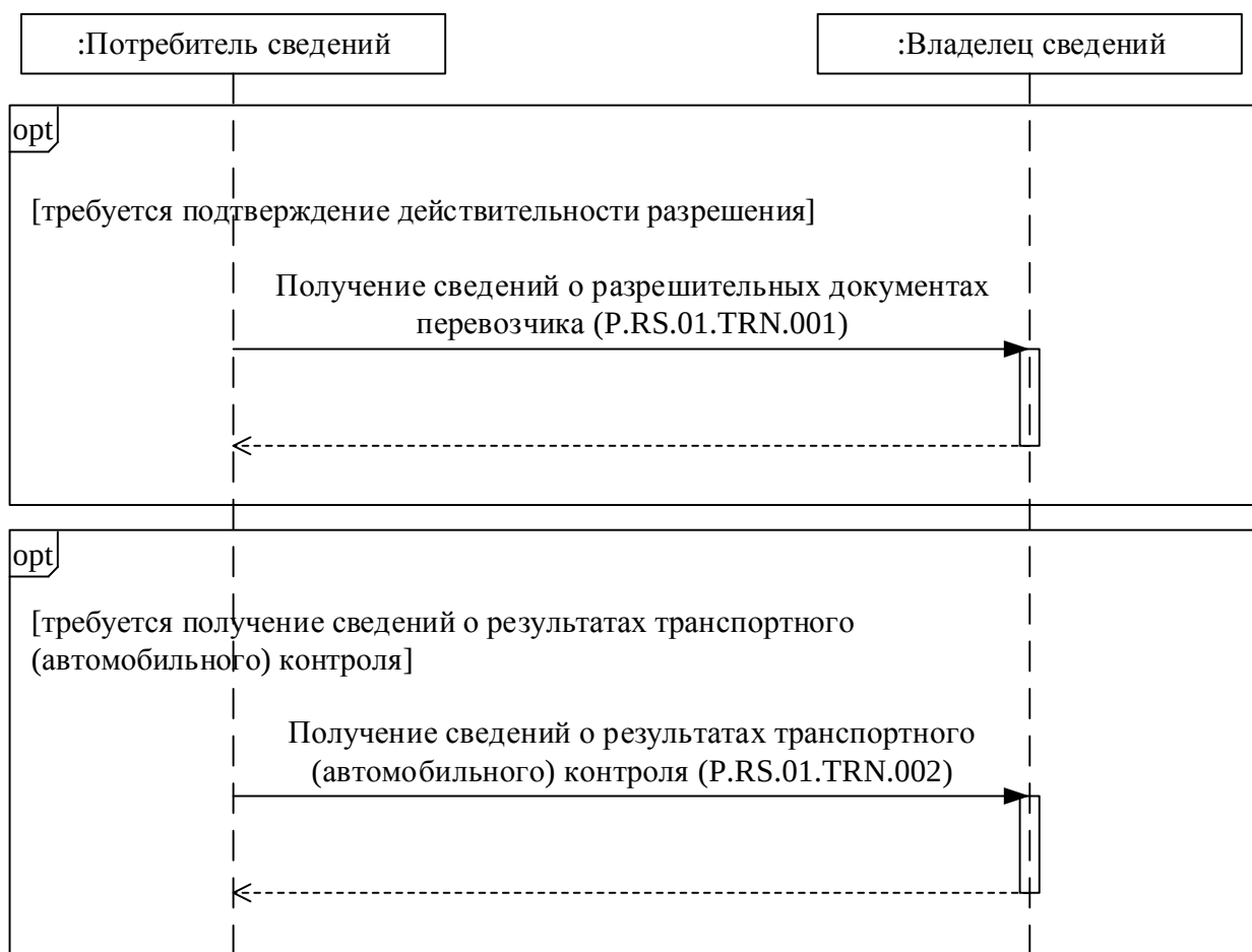
Рис. 2. Схема выполнения транзакций общего процесса при осуществлении транспортного (автомобильного) контроля
