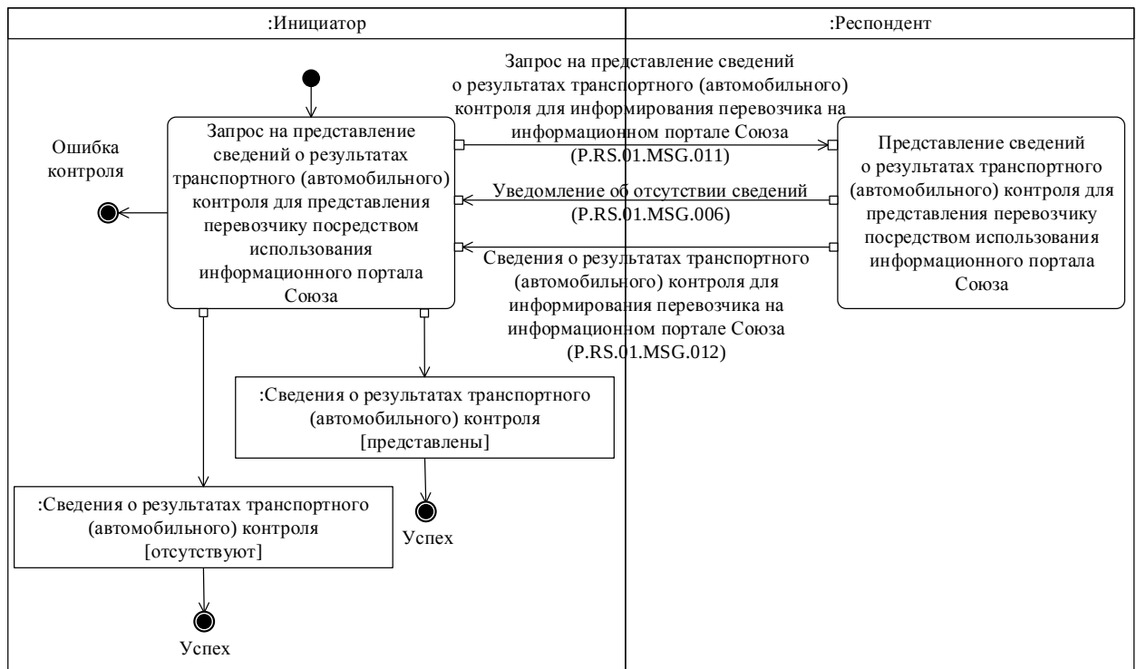
Рис. 3. Схема выполнения транзакции общего процесса «Получение сведений о результатах транспортного (автомобильного) контроля для представления перевозчику посредством использования информационного портала Союза» (P.RS.01.TRN.005)
