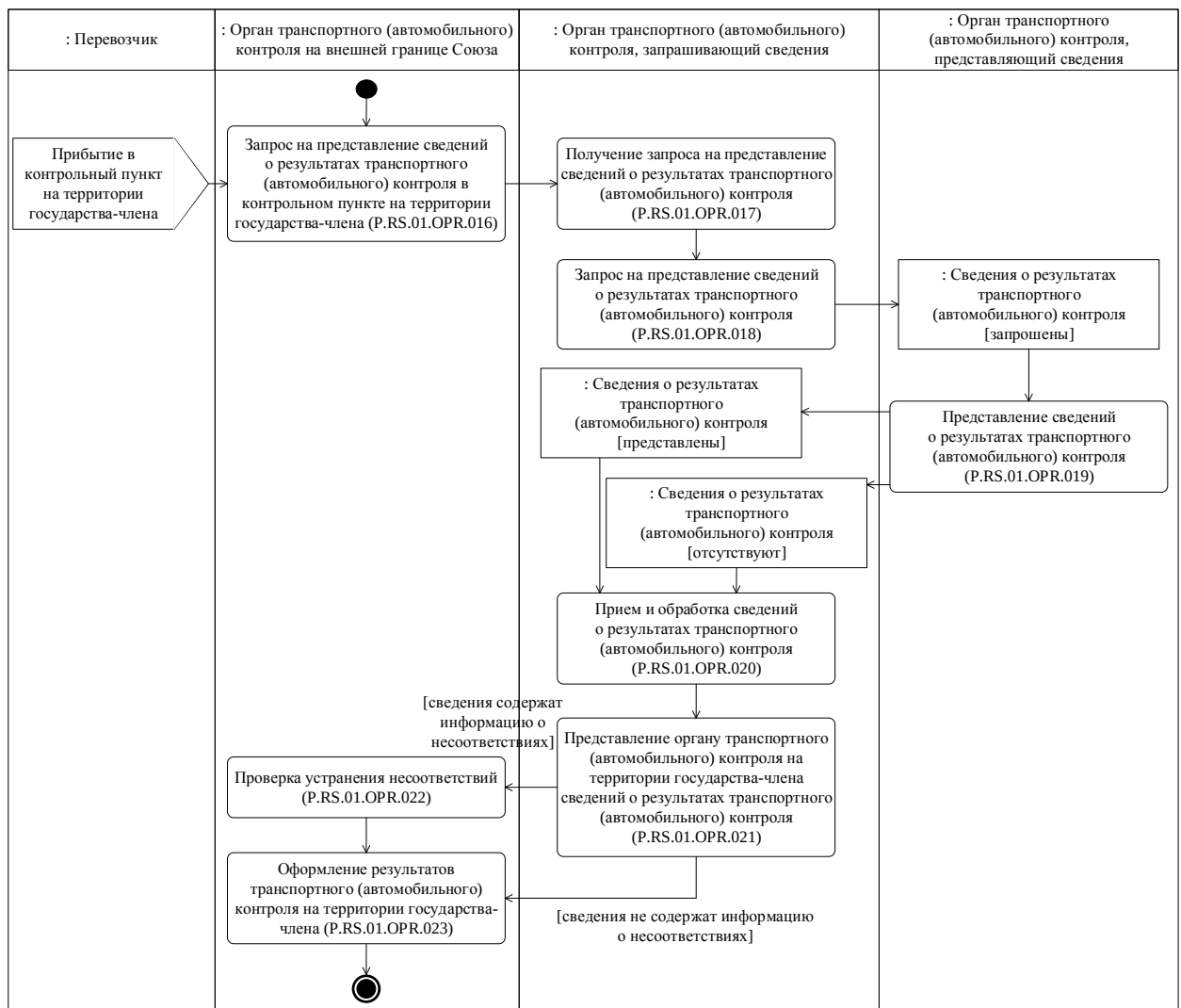
Рис. 6. Схема выполнения процедуры «Осуществление транспортного (автомобильного) контроля на территории государства-члена» (P.RS.01.PRC.002)
