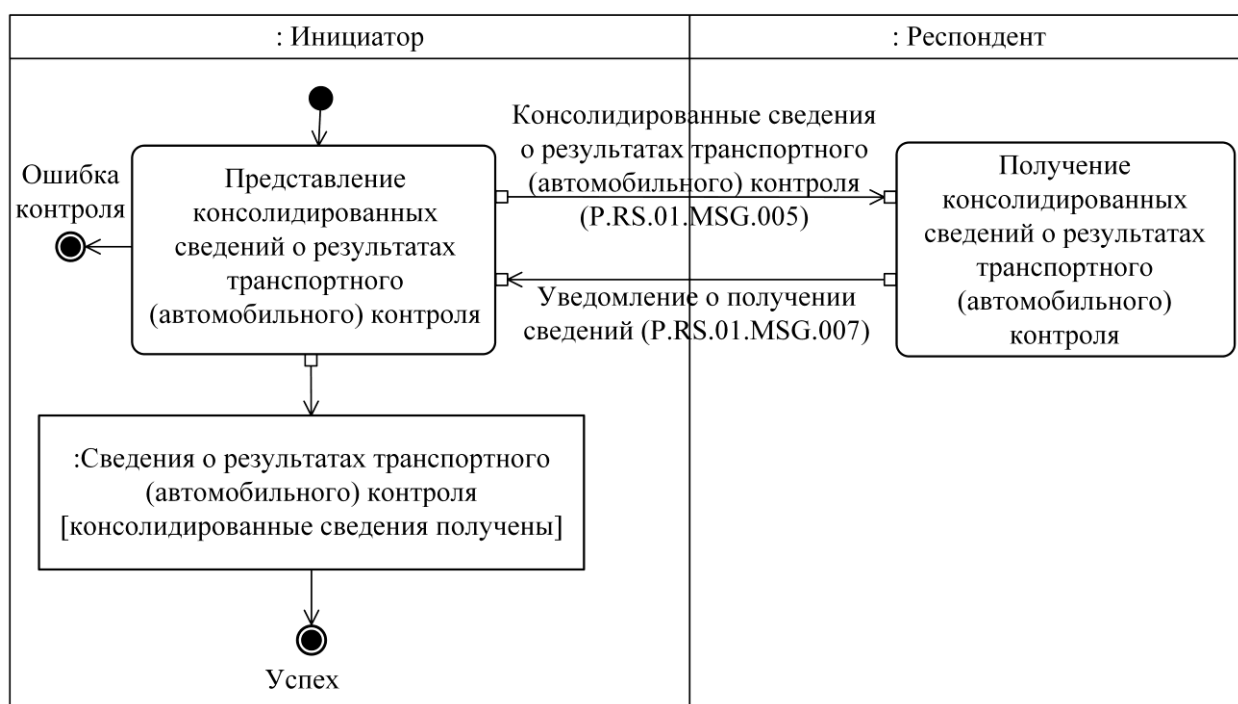
Рис. 7. Схема выполнения транзакции общего процесса «Передача консолидированных сведений о результатах транспортного (автомобильного) контроля» (P.RS.01.TRN.003)
