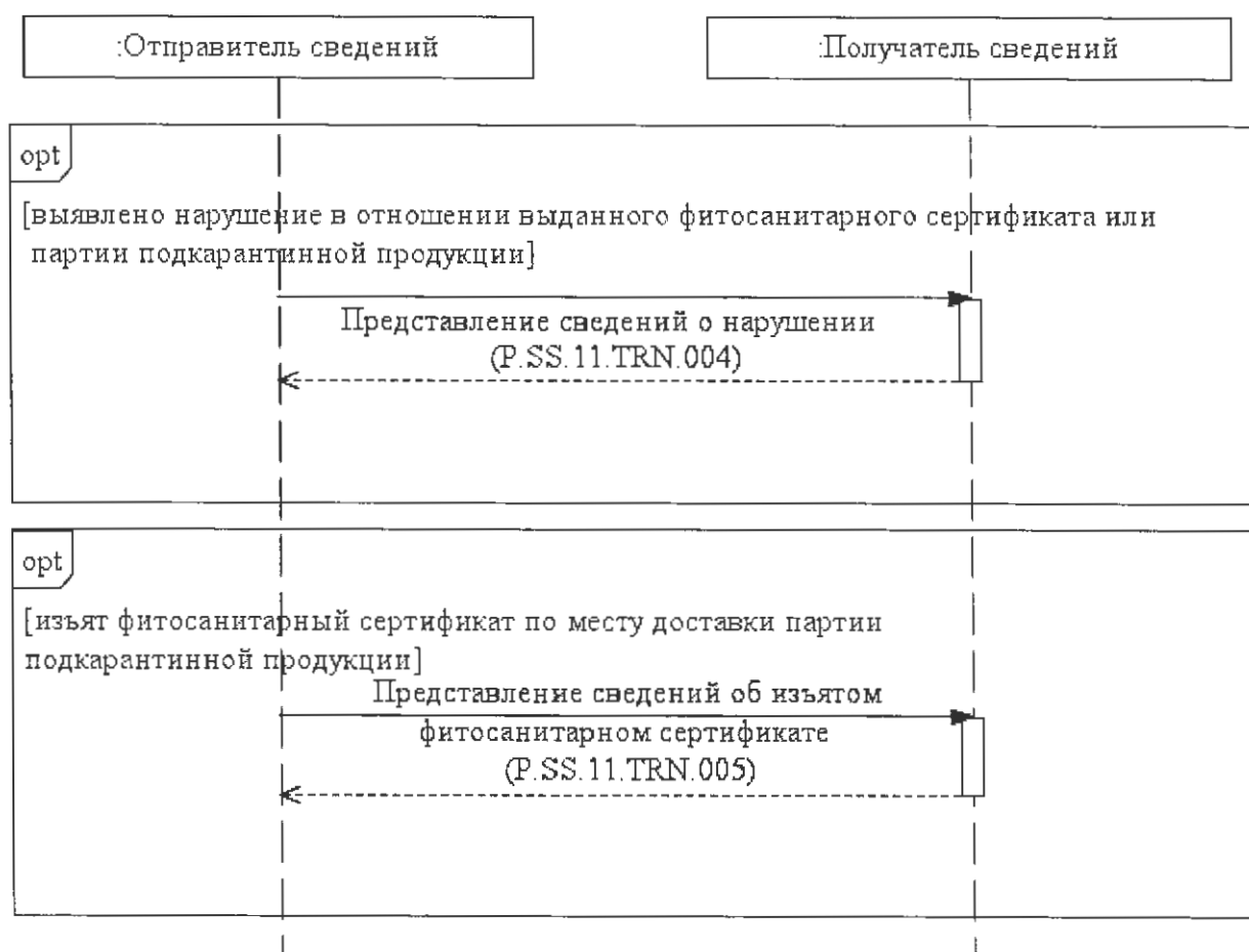
Рис. 3. Схема выполнения транзакций общего процесса при представлении сведений уполномоченному органу государства места отправления
