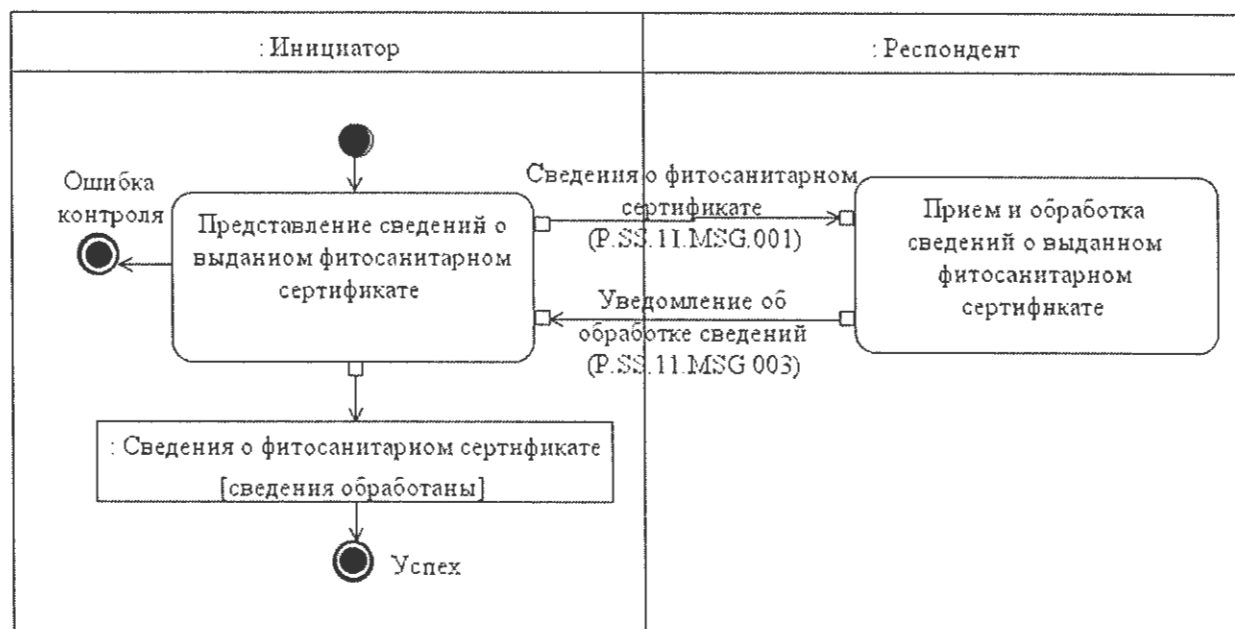
Рис. 5. Схема выполнения транзакции общего процесса «Представление сведений о выданном фитосанитарном сертификате» (P.SS.11.TRN.002)
