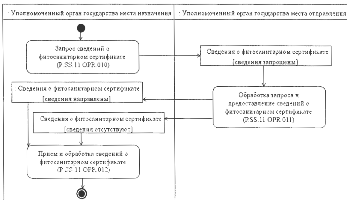
Рис. 5. Схема выполнения процедуры «Получение сведений о фитосанитарном сертификате по запросу» (P.SS.11.PRC.004)
