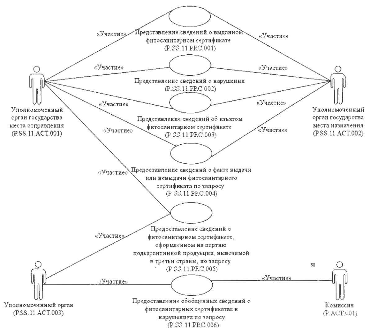
Рис. 1. Структура общего процесса
