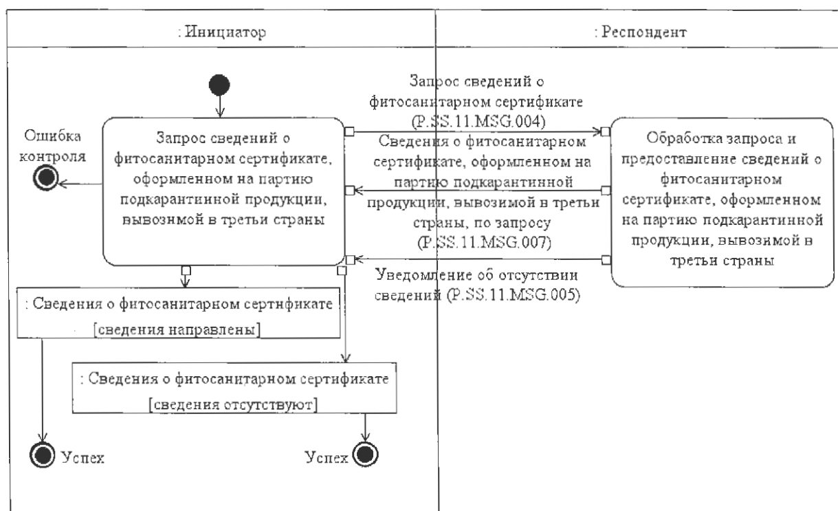
Рис. 9. Схема выполнения транзакции общего процесса «Предоставление сведений о фитосанитарном сертификате, оформленном на партию подкарантинной продукции, вывозимой в третьи страны» (P.SS.11.TRN.006)
