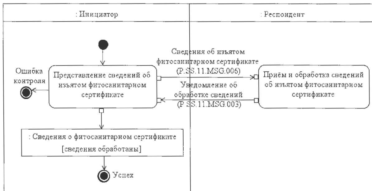
Рис. 8. Схема выполнения транзакции общего процесса «Представление сведений об изъятых фитосанитарных сертификатах» (P.SS.11.TRN.005)
