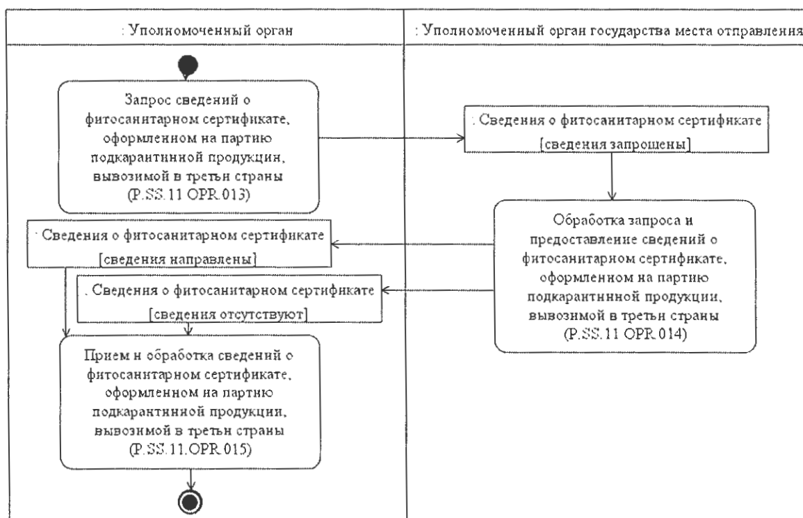
Рис. 6. Схема выполнения процедуры «Предоставление сведений о фитосанитарном сертификате, оформленном на партию подкарантинной продукции, вывозимой в третьи страны, по запросу» (P.SS.11.PRC.005)
