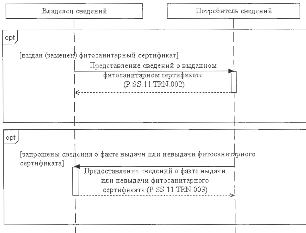
Рис. 2. Схема выполнения транзакций общего процесса при передаче сведений о выданном фитосанитарном сертификате
